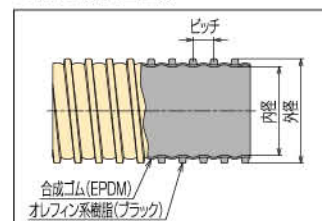
●構造(断面図)
