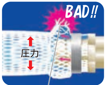
ホース膨張による 糸抜けパンク発生
